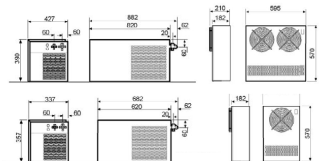
Parownik naścienny
